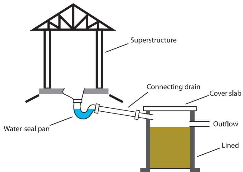
Fig A1.9: Pour and flush latrine
